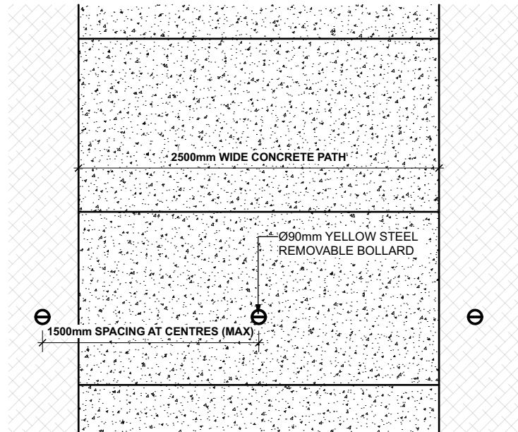
SETOUT : REMOVABLE BOLLARD SPACING
